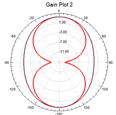
A-DA-A3035Antenna
